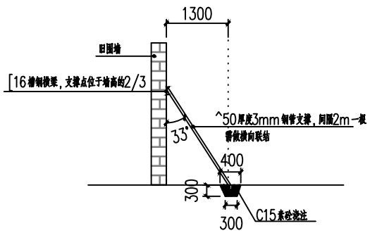
围墙1加固方案
